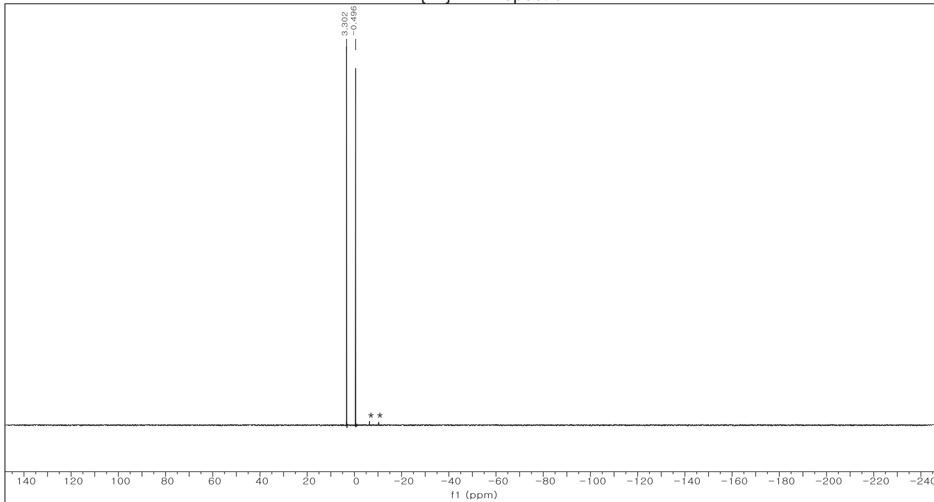
31 P{ 1 H} NMR spectrum
